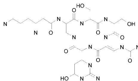
Viomycin
