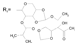
Evernimicin
