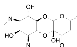
Viomycin
