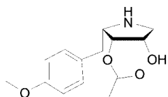
Anisomycin
