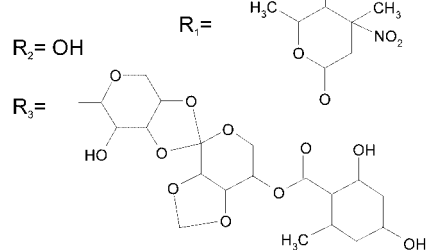
Evernimicin
