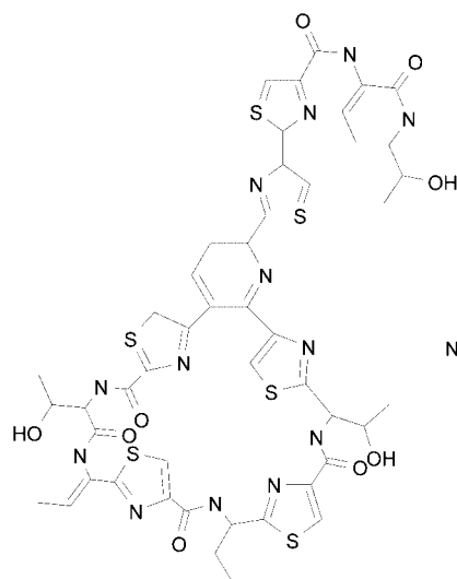
Micrococin
